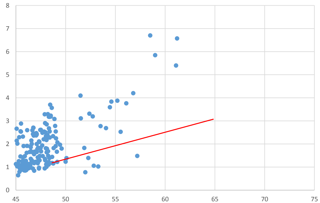
FeO*/MgO
