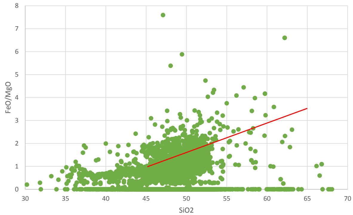
FeO/MgO vs. SiO 2
