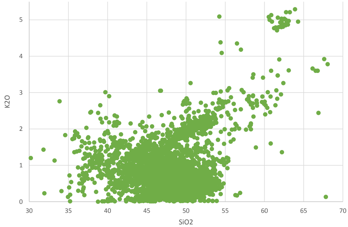
K2O vs. SiO2
