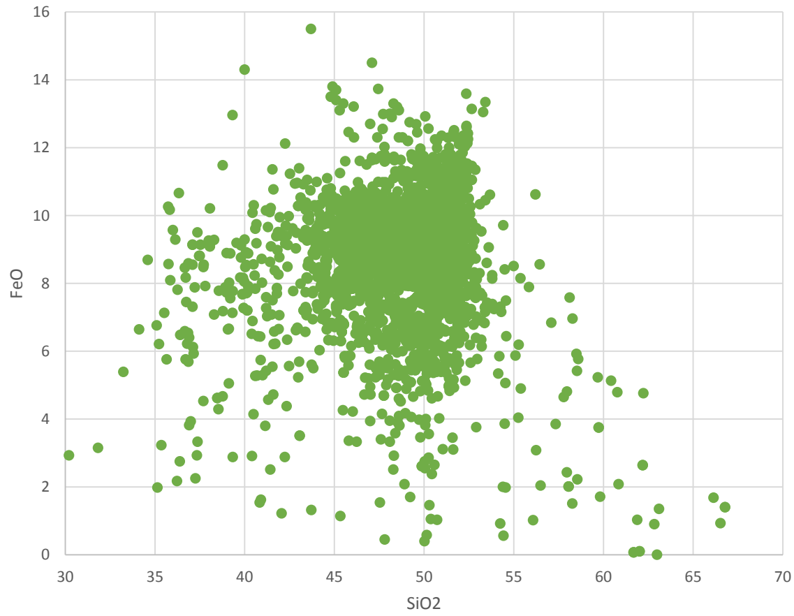
FeO vs. SiO2
