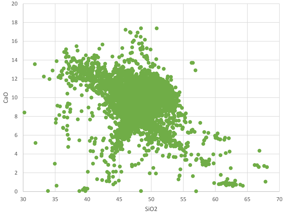
CaO vs. SiO2
