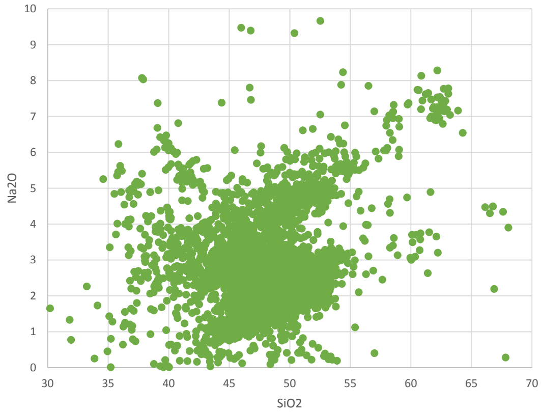
Na 2 O vs. SiO 2
