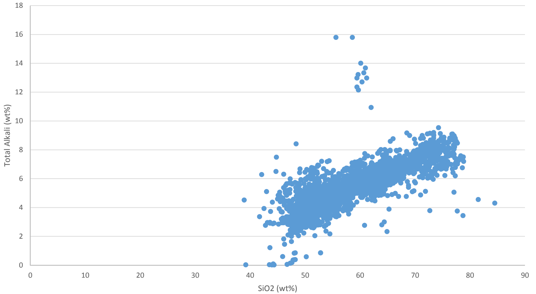
Total alkali vs. SiO2
